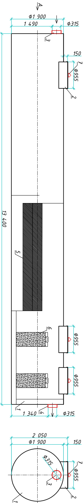
Разрез 1-1
